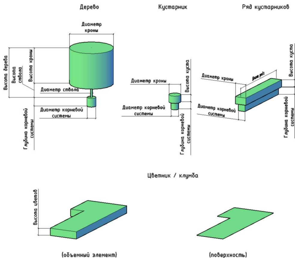
Рисунок 3.2.11 – Примеры выполнения элементов озеленения
